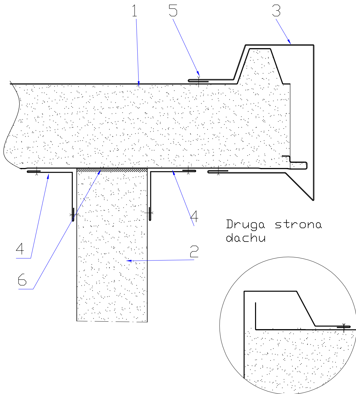
RYS. 19 POŁĄCZENIE PŁYT ŚCIENNEJ Z PŁYTĄ DACHOWĄ
